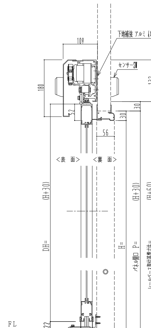
自動装置 Milion M-300AR
