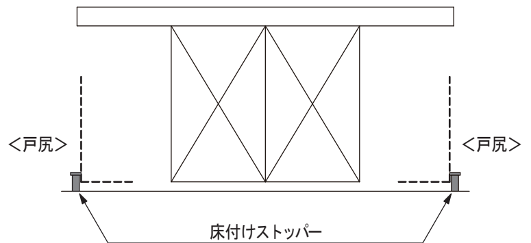
両引レール
