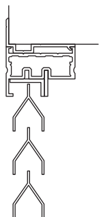
GAS-Y30 開口率=30%
