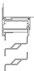
GAS-N52 開口率=52%
