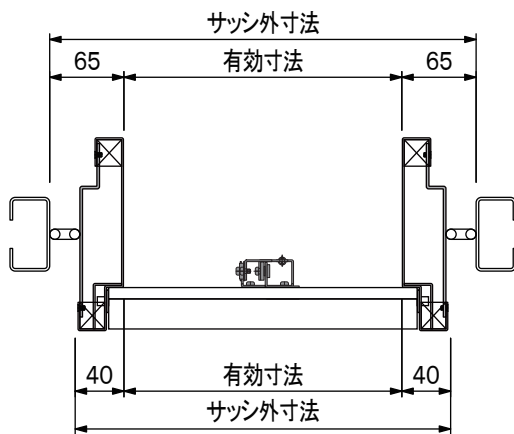
溶接固定
